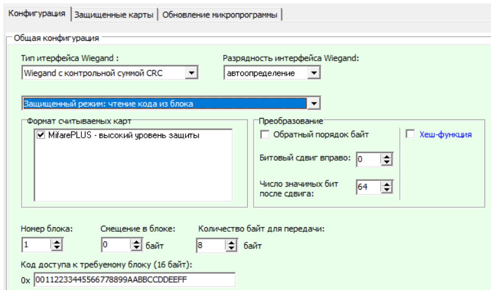
Рис. 3.6 Режим «чтение кода из блока»
