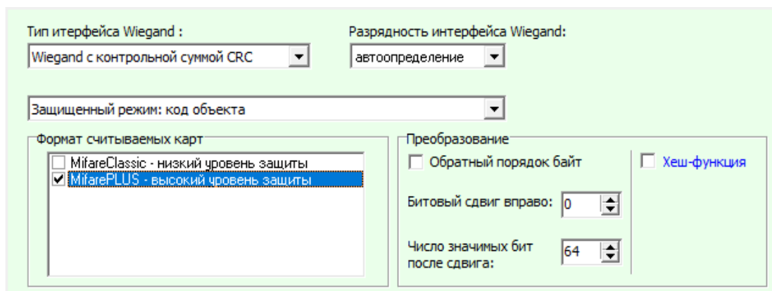
Рис. 3.1 Режим работы «код объекта»
