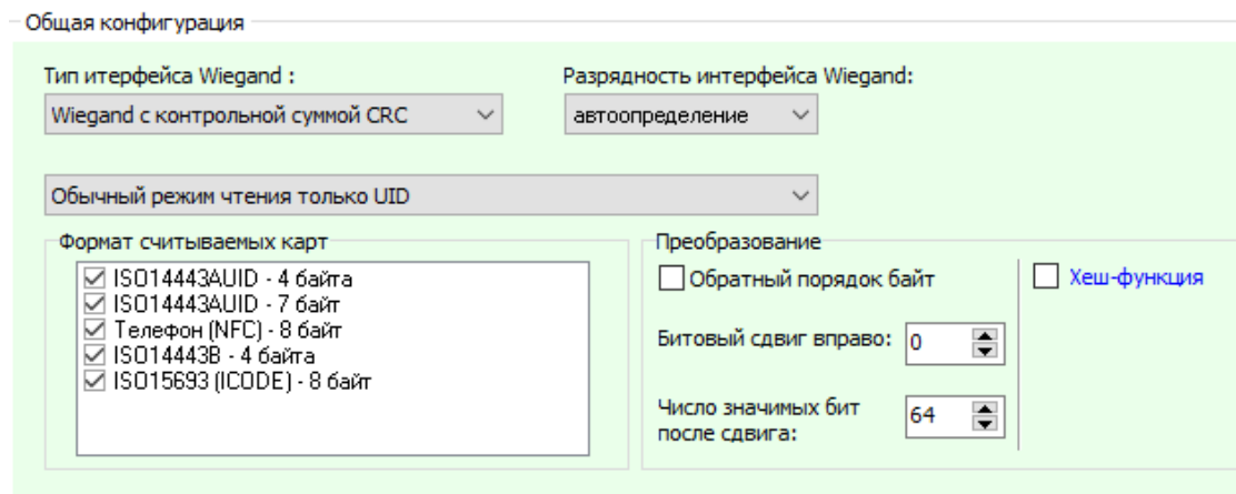
Рис. 2.5 Настройки по умолчанию
