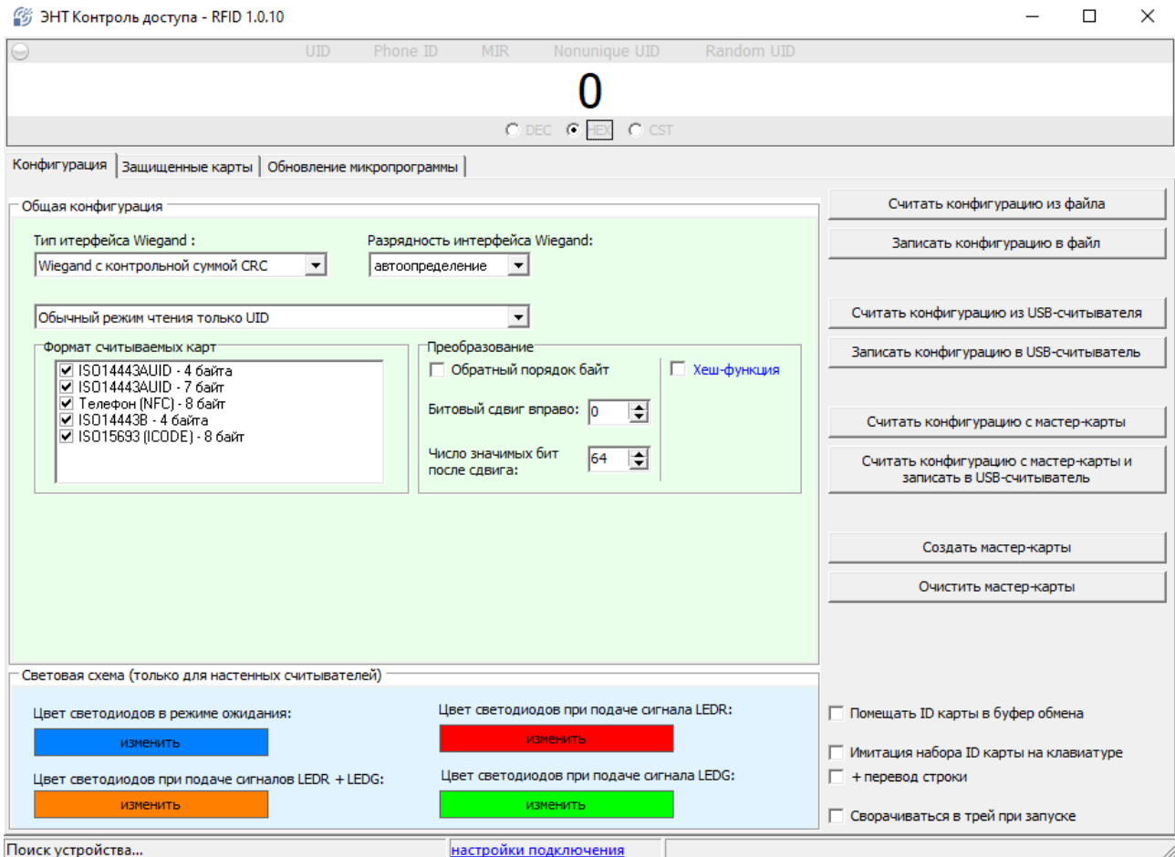
Рис. 2.1 Внешний вид программы
