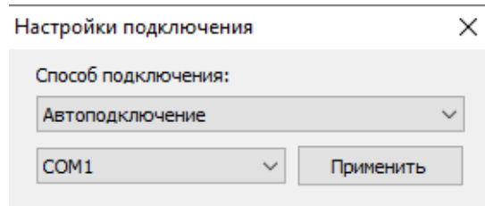
Рис. 2.4 Настройки подключения
